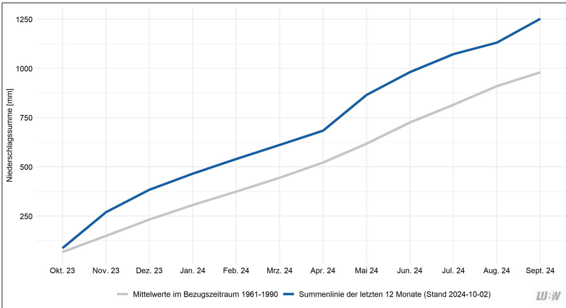
Abbildung 2: Summenlinie des Niederschlags in den vergangenen Monaten in Baden-Württemberg im Vergleich mit dem Referenzzeitraum 1961-1990.
