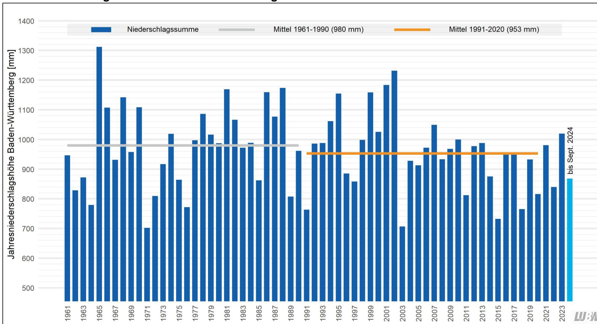
Abbildung 3: Jahresniederschlagshöhen in Baden-Württemberg seit 1961. Die mittlere Jahresniederschlagshöhe in den Vergleichszeiträumen 1961-1990 (grau) und 1991-2020 (orange) sind ebenfalls eingezeichnet.
