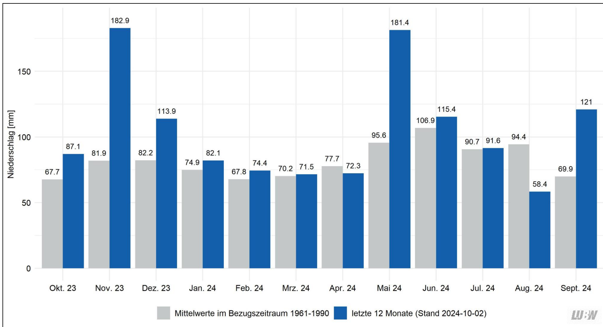
Abbildung 1: Niederschlag in den vergangenen Monaten in Baden-Württemberg im Vergleich mit den Mittelwerten im Referenzzeitraum 1961-1990.
