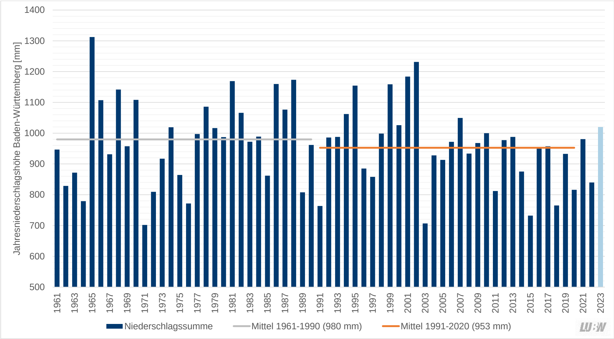
Abbildung 2: Jahresniederschlagshöhe in Baden-Württemberg im Zeitraum 1961 bis 2023 (Stand 03.01.2024). Die mittlere Jahresniederschlagshöhe in den Vergleichszeiträumen 1961-1990 (grau) und 1991-2020 (orange) sind ebenfalls eingezeichnet.
