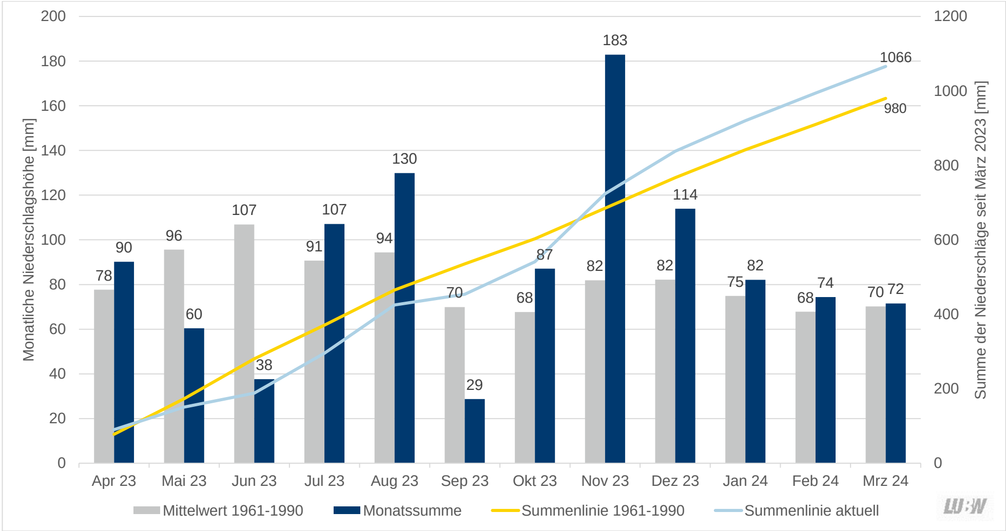
Abbildung 1: Niederschlag in den vergangenen Monaten in Baden-Württemberg im Vergleich mit den Mittelwerten im Referenzzeitraum 1961-1990.
